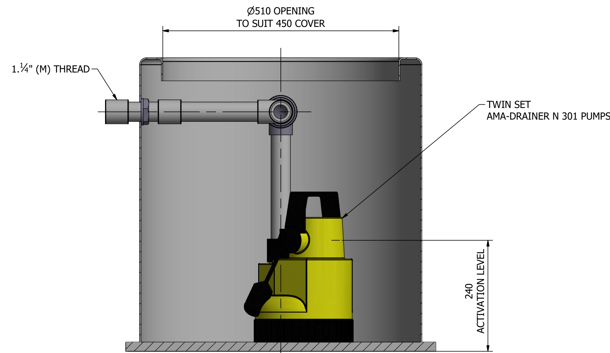
SECTION A-A SCALE 1:5
