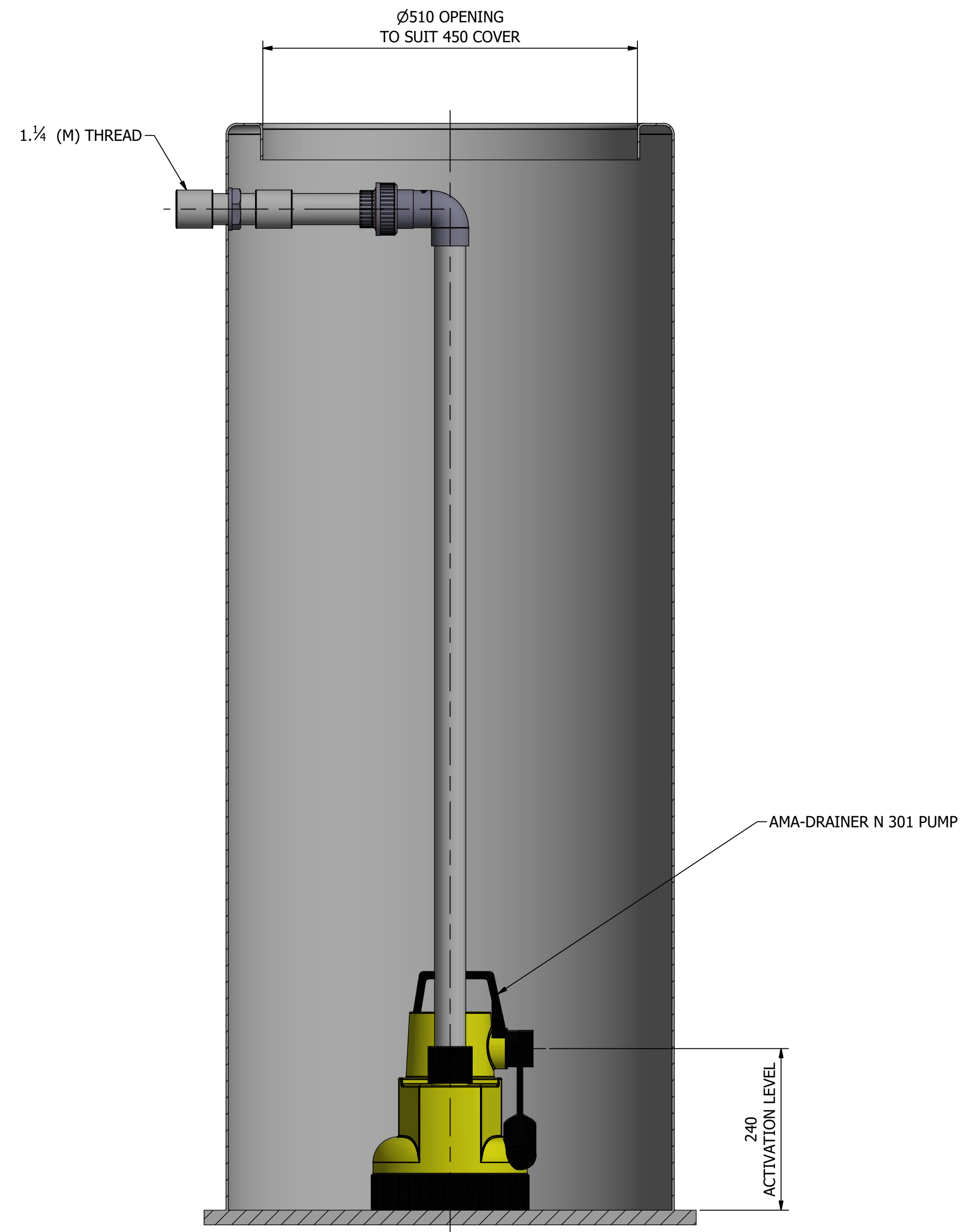
SECTION A-A SCALE 1:5
