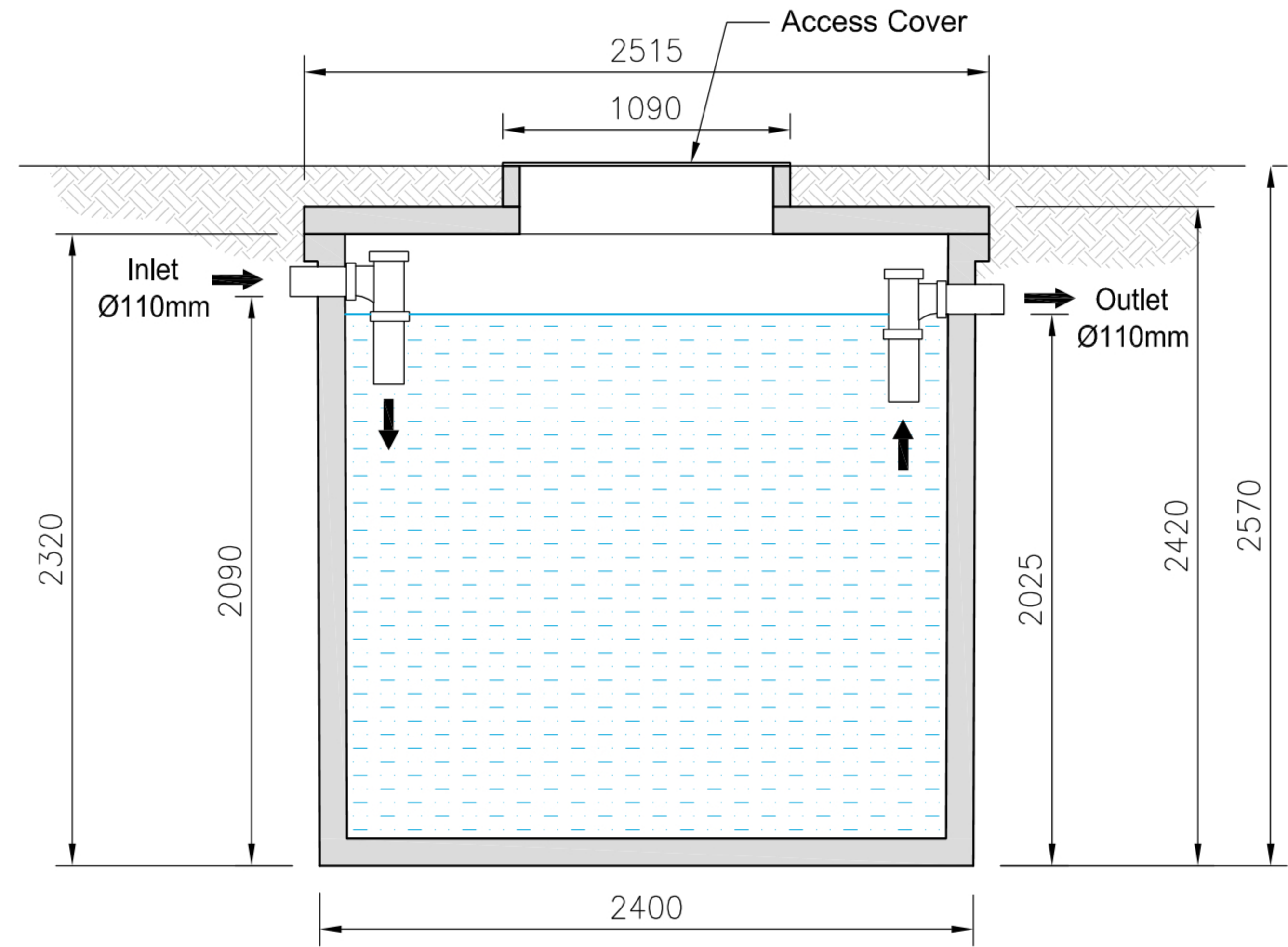
Section A-A
