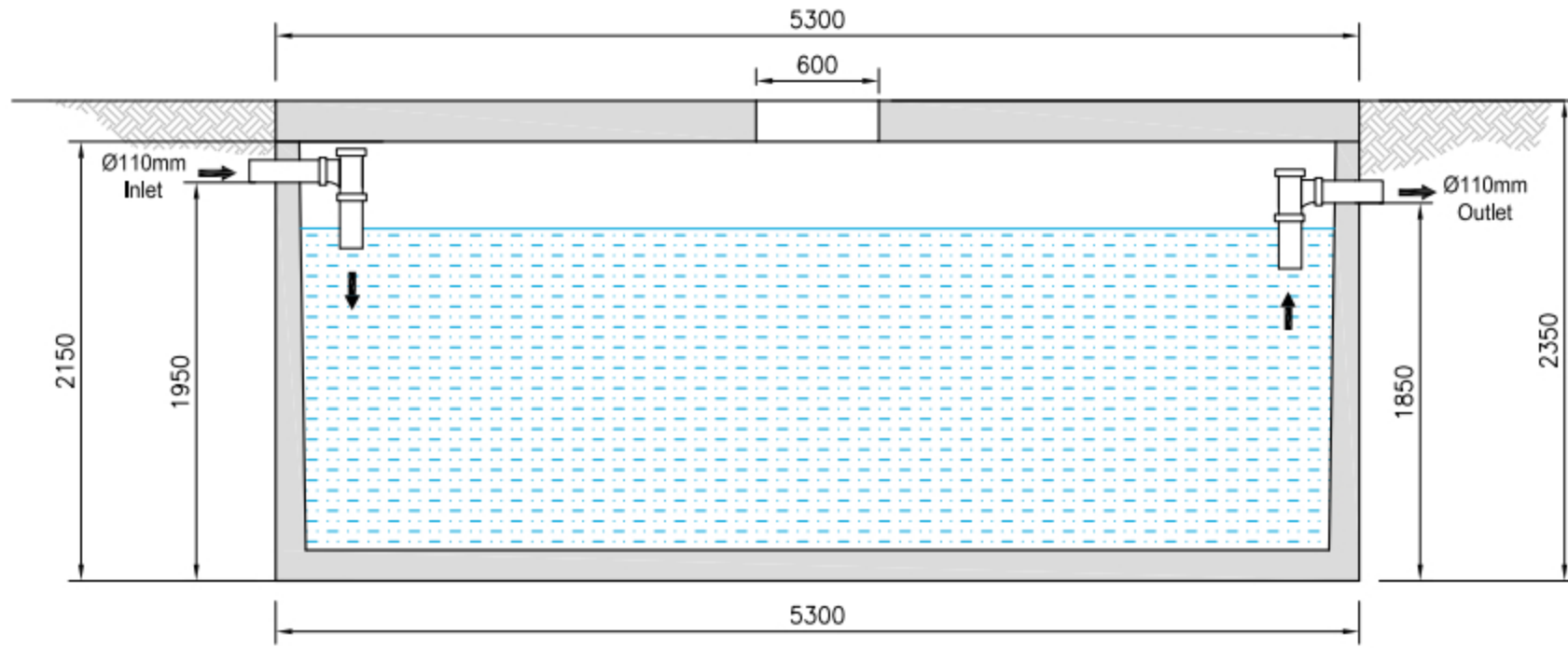
Section A-A
