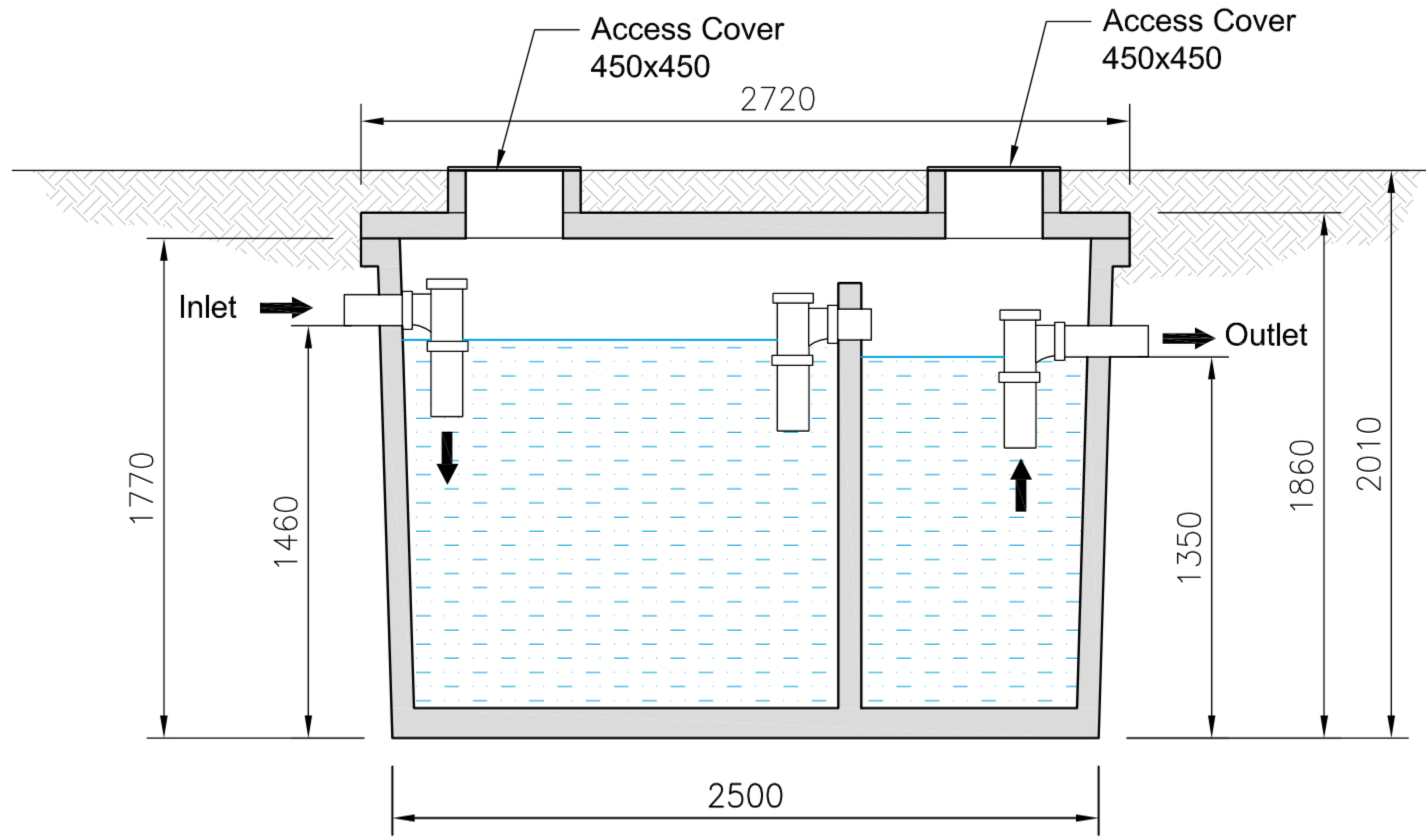
Section A-A
